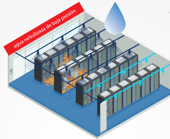
Agua nebulizada baja presión (LPWM)
